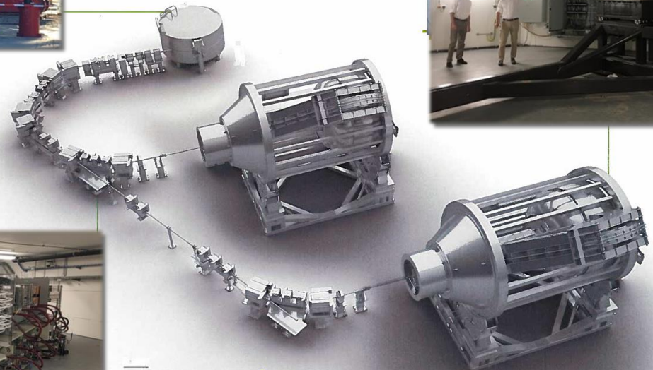
Gantry 10 meter 100 ton
